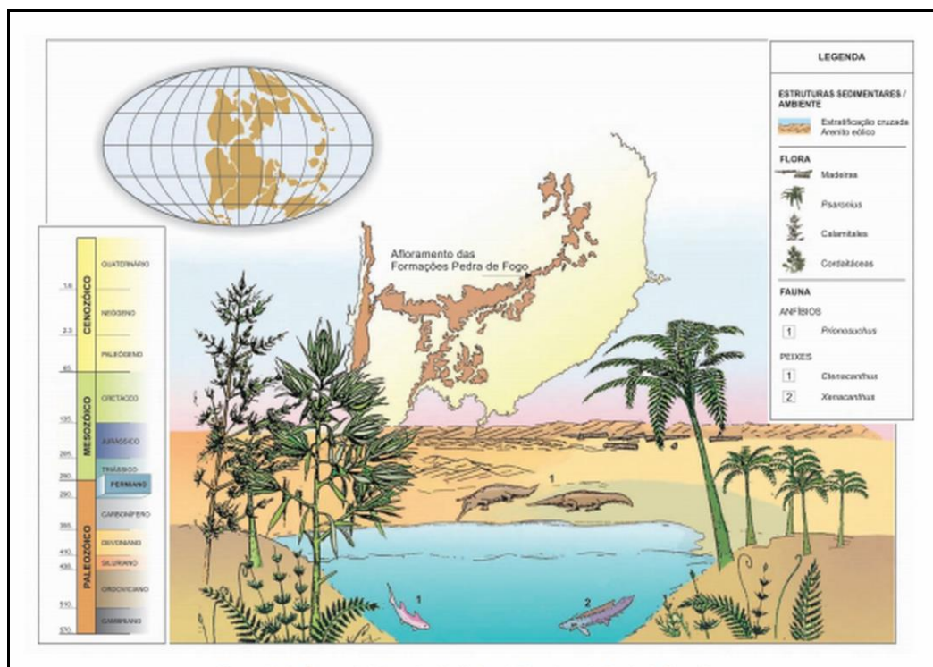
Figura 02 – Formação Pedra de Fogo no Brasil
