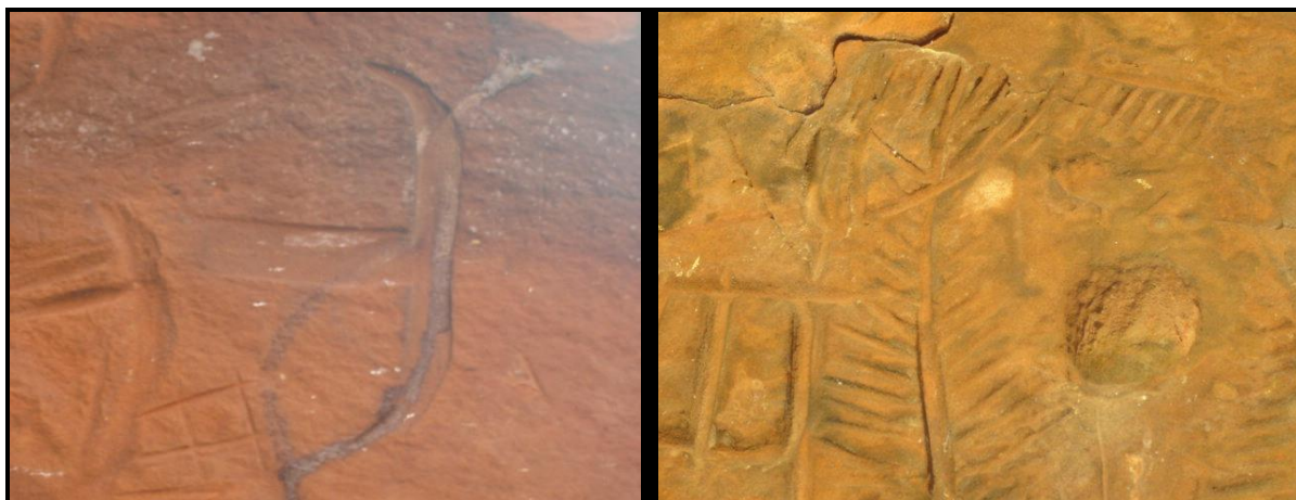
Figura 08 – Inscrições Rupestres em Arenito Eólico
